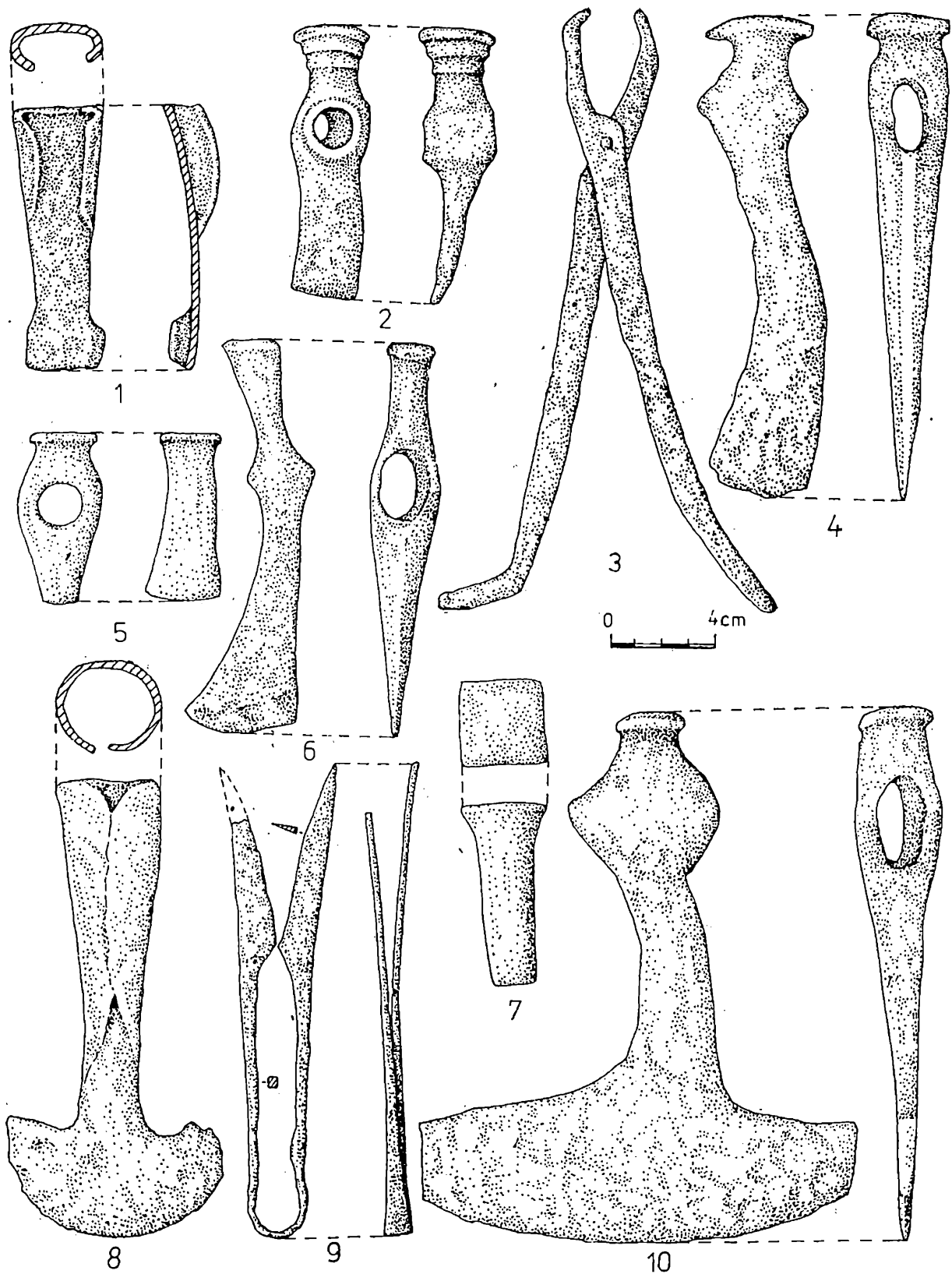
Fig. 9. — Unelte din fier din secolele VIII—X e.n. 1, Fundu-Herții; 2, Mateeni; 3, Suletea; 4, Hangu; 5, 7, Dragosloveni; 6, Fedești; 8, Floreni; 9, Dodești; 10, Tăvădărești.
