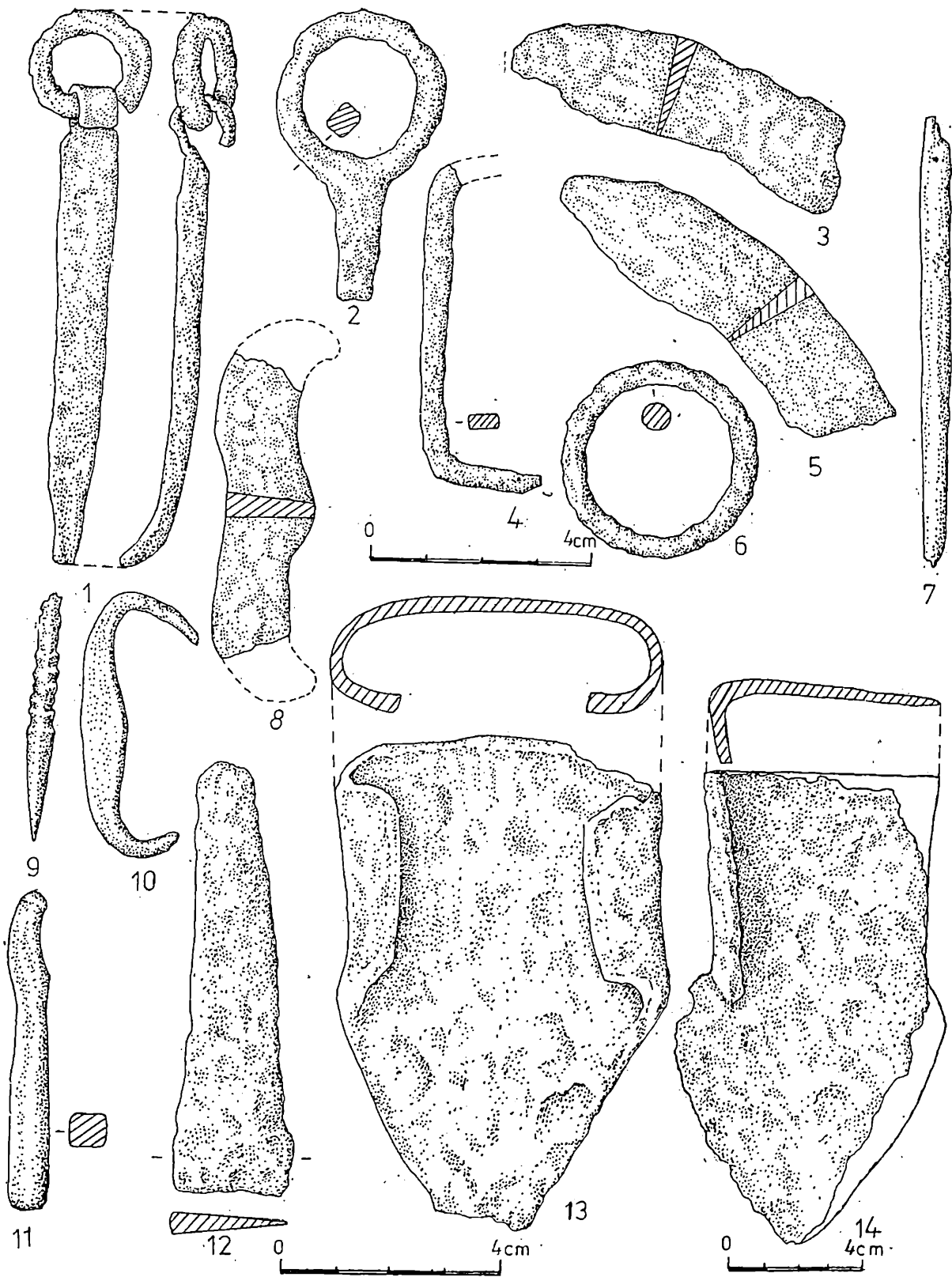
Fig. 2. — Unelte din secolele V–VII c.n. 1, 4, 7, 9–13, Dodești; 2–3, 6, 8, Botoșana; 5, Davideni; 14, Buțuluc.
