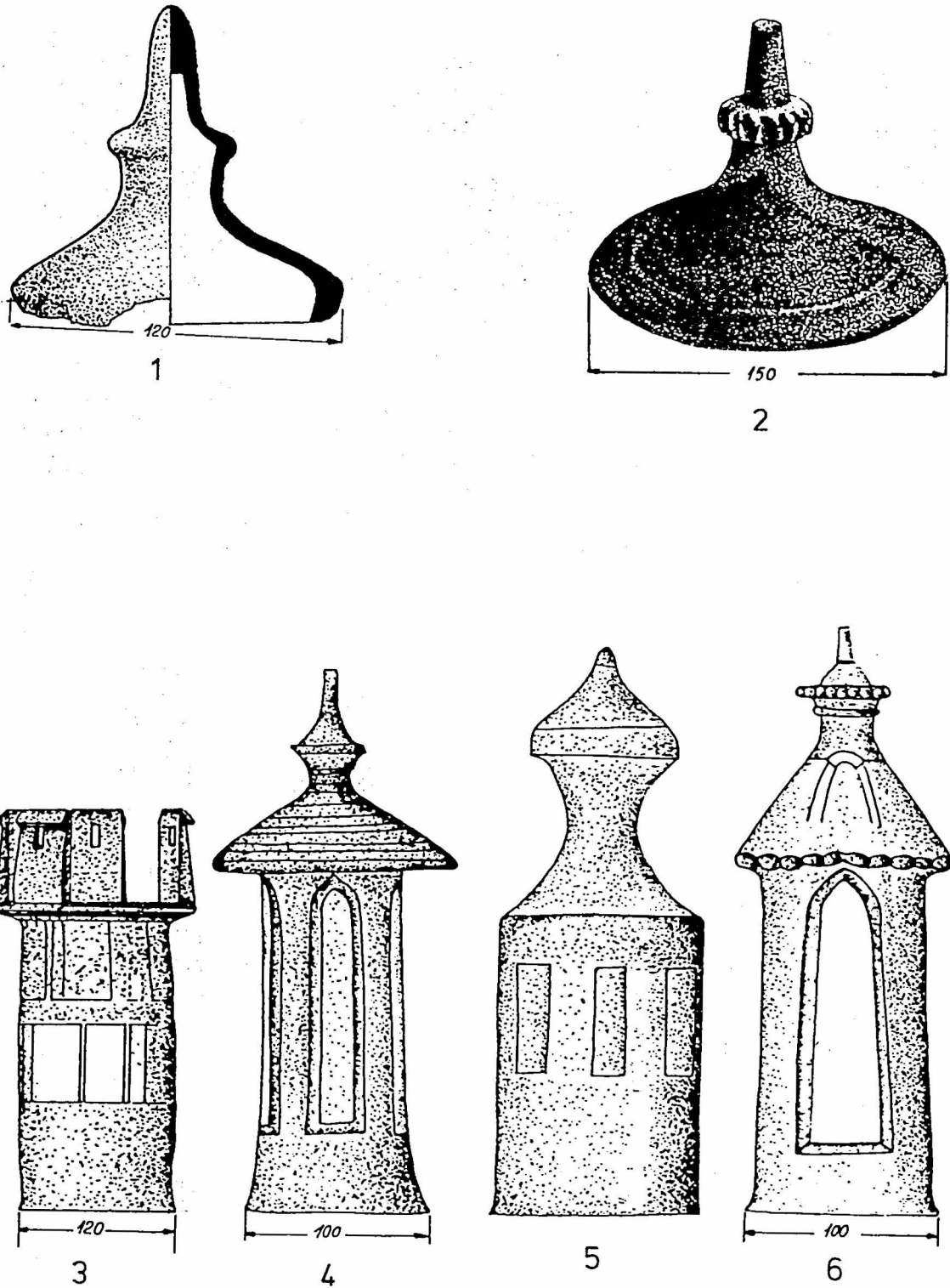
Fig. 12. Fragmente de cahle (1-2) și cahle-turn (3-6) descoperite la Suceava (1-3), vechea mănăstire Humor (4, 6), Orheiul Vechi (5), după R. Popa, M. Mărgineanu-Cârstoiu (3), E. Busuioc, M. Mărgineanu-Cârstoiu (4, 6), G. D. Smirnov (5).
