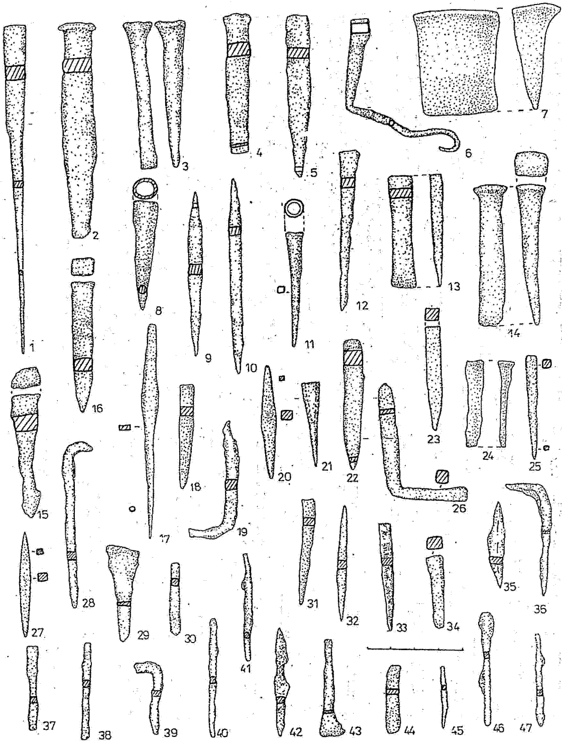
Fig. 15. Poiana. Dornuri (2, 5, 15-16, 22, 25, 34), străpungători (1, 6, 8-12, 17-18, 20-21, 23, 27-29, 31-33, 35, 40-42, 45); dălți (3-4, 13-14, 24, 43), nicovală (7), scoabe (19, 26, 36-37, 39), cui (30) și bare (38, 44, 46-47) de fier.
