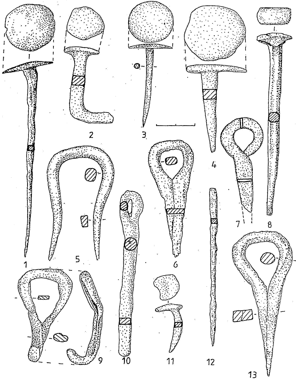
Fig. 24. Poiana. Piroane (1-2, 4, 8), cuițe (3, 11), împungător (12), tățâni (6, 9, 13), scoabă (5), incuicloare (7) și bară (10) de fier și bronz (3).
