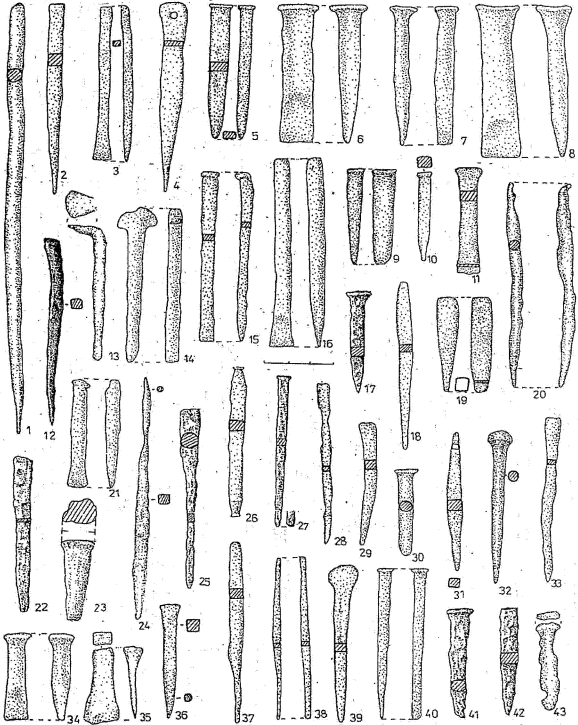
Fig. 14. Poiana. Dălți (3-4, 6-9, 11, 15-16, 19, 21, 27, 34-35, 40), străpungători (1-2, 12, 18, 20, 22, 24, 28-29, 31, 33, 37-38), domuri (5, 10, 17, 23, 25-26, 30, 32, 36, 39, 41-43) și cuie (13-14) de fier.
