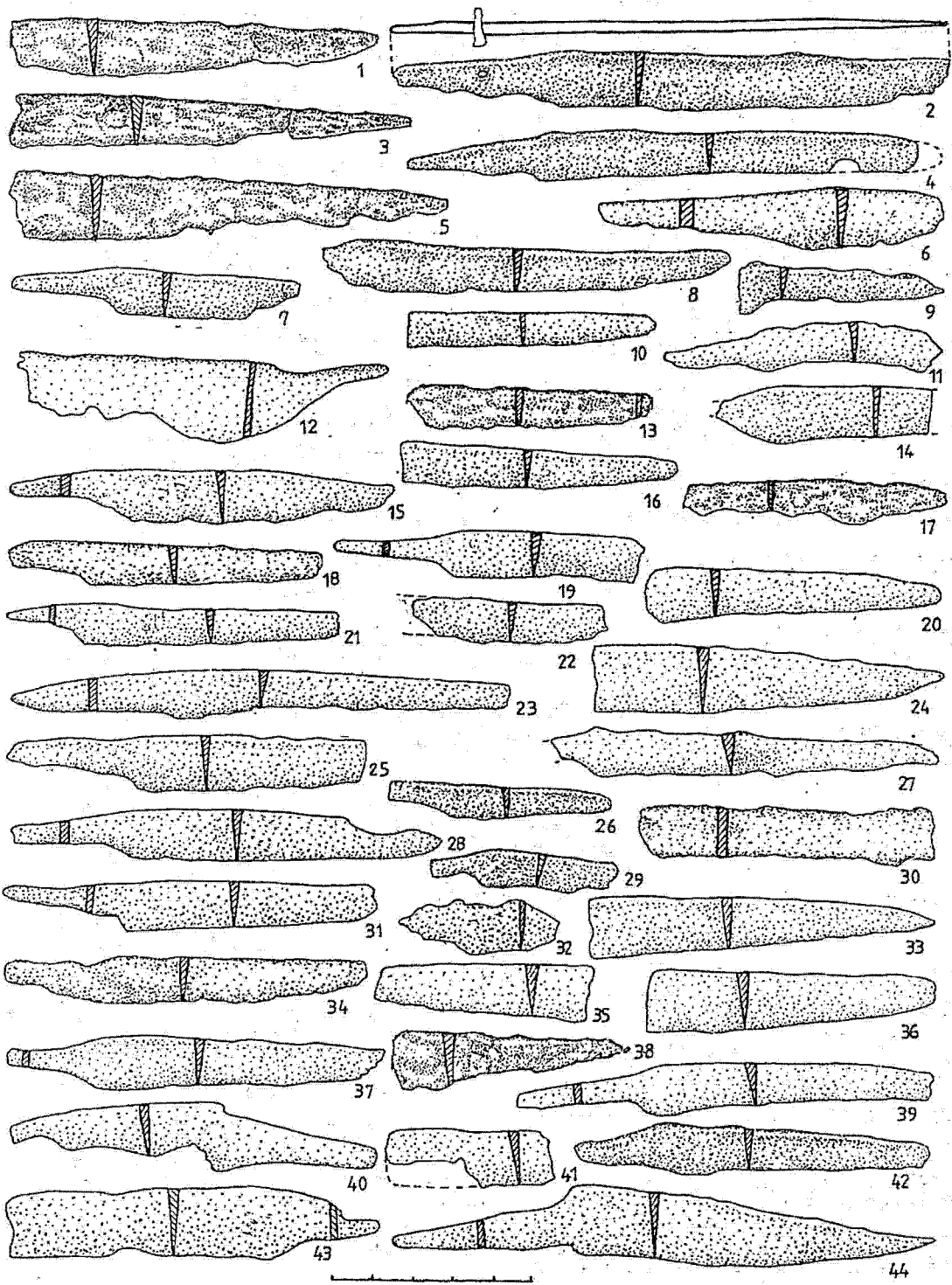
Fig. 9. Poiana. Cujite (1-44) de fier.
