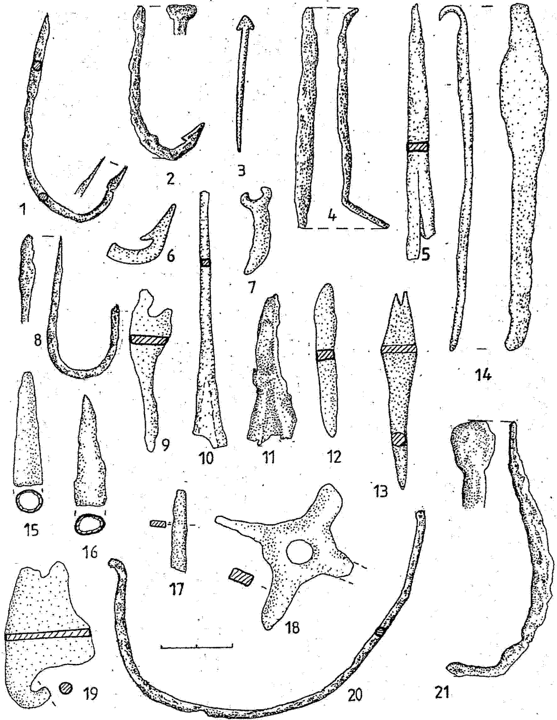
Fig. 23. Poiana. Cârlige de undiță (1-2, 6, 8, 21), împungători (3, 5, 12, 15-16), scoabe (4, 17), paletă (9), elice (18), mâner (19-20), vârfuri (7, 10-11, 14) și daltă (13) de fier.
