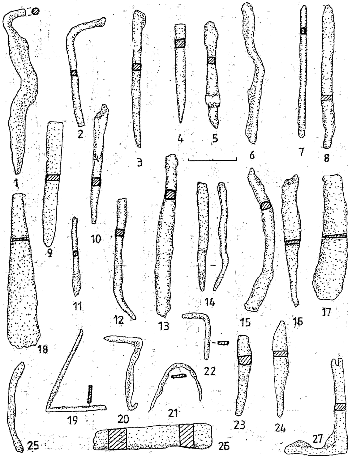
Fig. 18. Poiana. Scoabe (1-2, 4, 10-12, 14, 19, 22, 24-25), străpungători (3, 23), cui (11), pila (16), cuțit (17), daltă (9), fragmente de tablă (18, 20-21) și diferite bare (5-8, 13, 15, 27) de fier.
