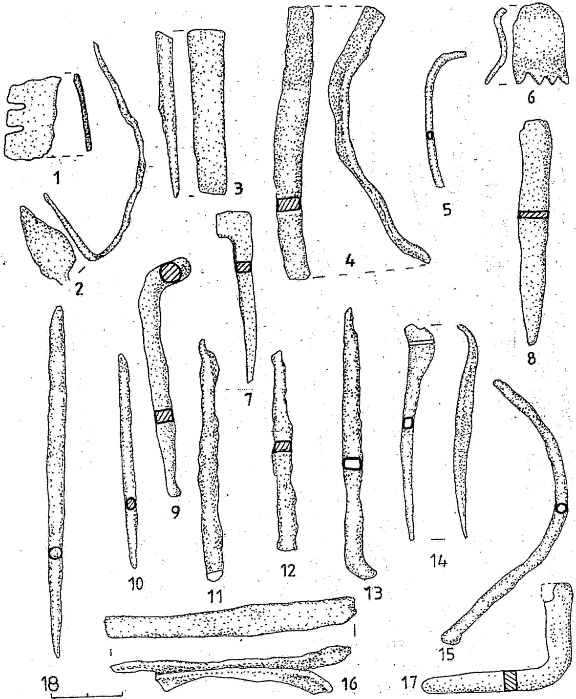
Fig. 19. Poiana. Fragmente de tablă (1, 6, 16), spatulă (2), daltă (3), sârmă (5, 15), pilă (8), scoabe (7, 13-14, 17), străpungători (10, 12, 18) și bare (4, 9, 11) de fier.
