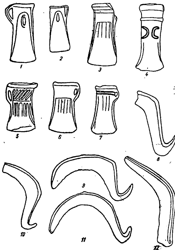
Fig. 6. — Obiecte de bronz descoperite izolat la : 1 — Bogdana ; 2 — Dănești ; 3 — Bunești ; 4 — Emil Racoviță ; 5 — Tg.-Neamț. 6 — Scheia, raionul Negrești ; 7 — Preușești ; 8 — Ciurești ; 9 — Boureni ; 10 — Broscăuți ; 11 — Cîrja ; 12 — Scheia, raionul Suceava (1-3, 6-10, 12 = 1/2 ; 4-5, 11 = 1/3).
