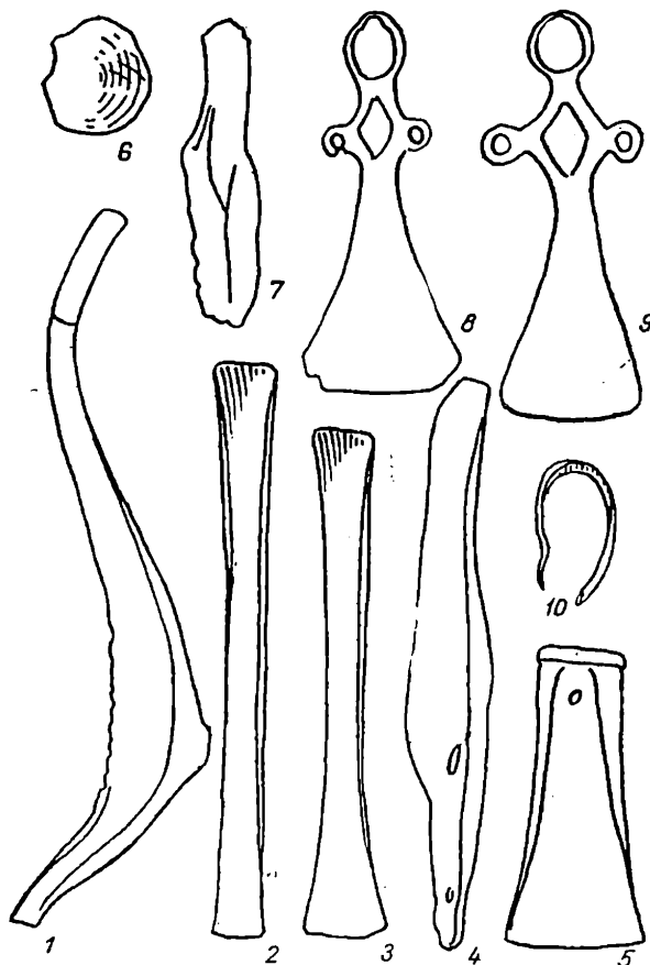
Fig. 5. — Depozitul de obiecte de bronz de la Ulmi-Liteni (1 - 10 = 1/2).
