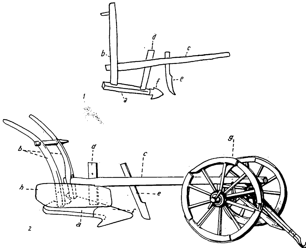
Fig. 5. - Unelte de arat cu plaz: 1 - aratru; 2 - plug; a - plaz; b - coarne; c - grindei; d - birsă; e - cuțit; f - brazdar; g - cotigă; h - cormană.
