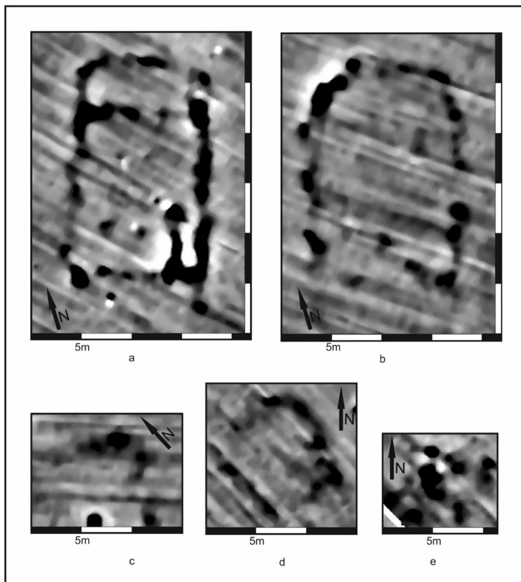
Fig. 2. Structuri vizibile în scanarea geomagnetică, identificate în interiorul fortificației.
