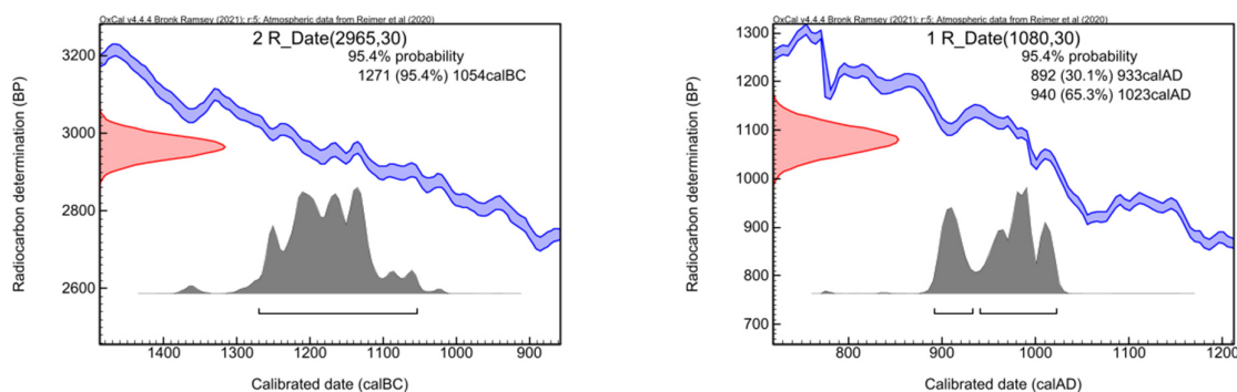
Fig. 4. Datele radiocarbon de la Drăgușeni – Dealu' Chițanca calibrate.
