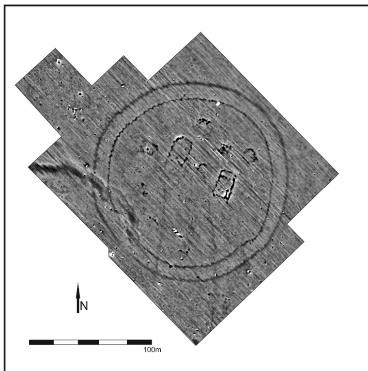
Fig. 1. Scanarea geomagnetică a fortificației de la Drăgușeni – Dealu' Chițanca.
