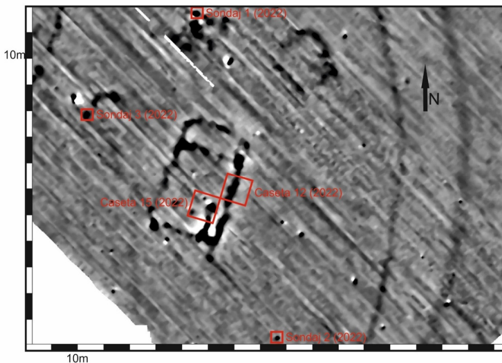
Fig. 3. Poziționarea unităților de cercetare pe Structura 1 și Sondajele 1 și 3, efectuate pe Structurile 4 și 6. Sondajul 2 efectuat pe o anomalie geomagnetică.
